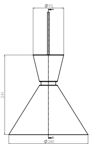
Ø 24cm
