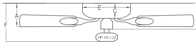
VENTILADOR DECORATIVO
