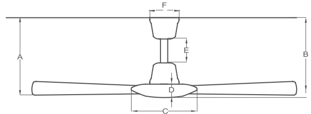
VENTILADOR INDUSTRIAL
